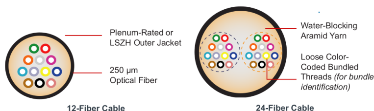
12-Fiber Cable
