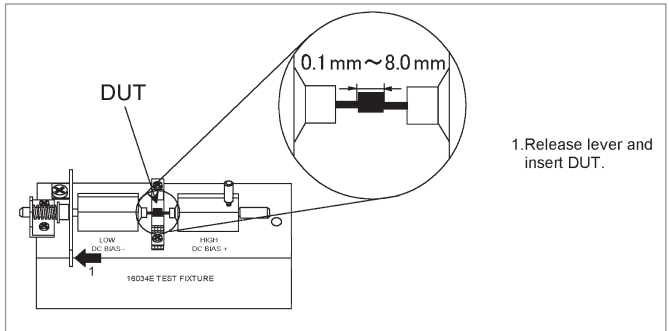
Inserting a DUT
