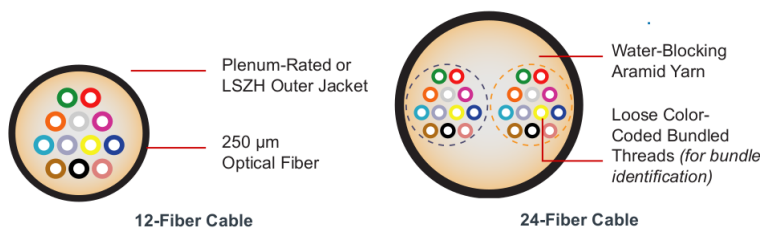
12-Fiber Cable
